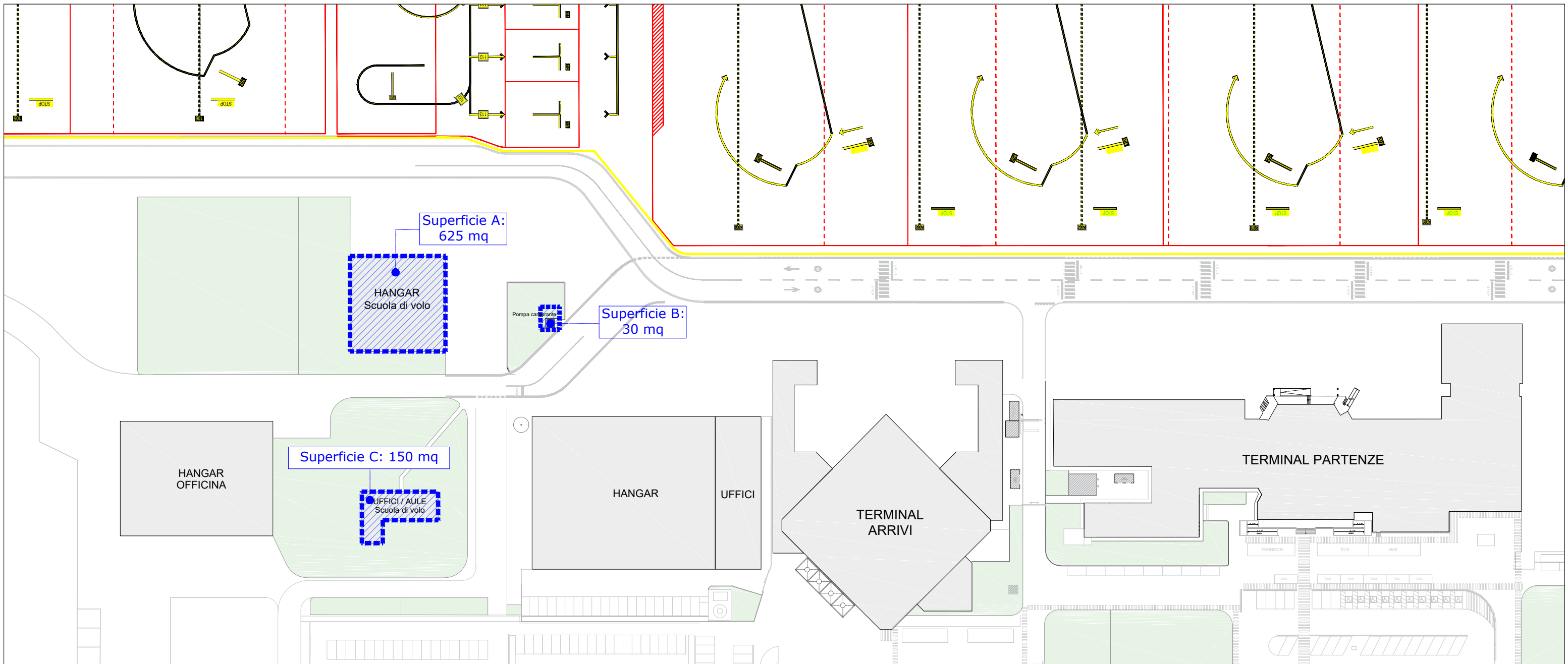
Aree scuola di volo _Scala 1:100
